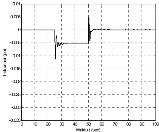
Gambar 12. Hasil simulink kendalian menggunakan governor fuzzy logic dengan perubahan beban 0,5 pu
