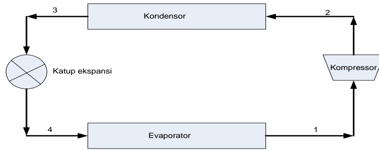
Gambar 1. Komponen utama dari mesin refrigerasi
