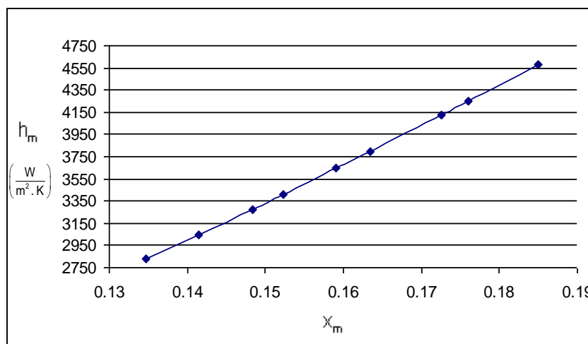
Gambar 3. Grafik hubungan koefisien perpindahan panas rata-rata dengan kualitas uap rata-rata
