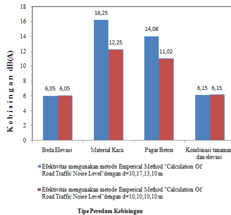
Gambar 7 Perbandingan efektivitas empirical method ( calculation of road noise level ) pada jarak yang bervariasi dan sama
