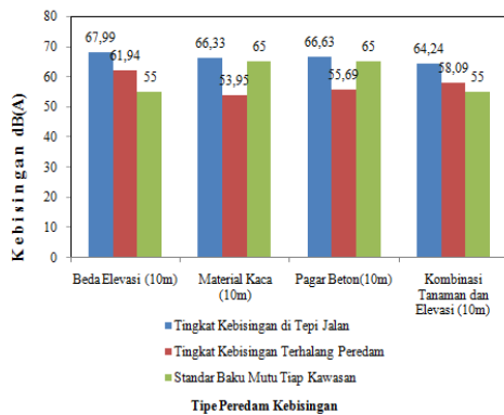
Gambar 5. Hubungan tingkat kebisingan berbagai tipe peredam pada jarak sama dengan Standard Baku mutu menggunakan empirical method menggunakan "Calculation of Road Noise Level"
