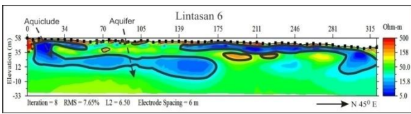
Gambar 9. Pemodelan Penampang 2D Lintasan 6
