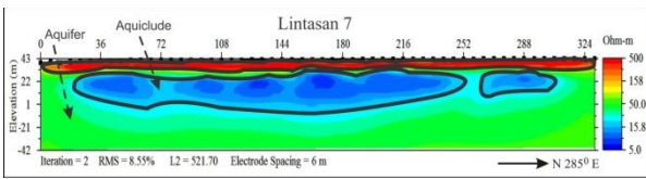
Gambar 10. Pemodelan Penampang 2D Lintasan 7
