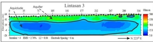
Gambar 6. Pemodelan Penampang Lintasan 3
