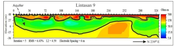
Gambar 12. Pemodelan Penampang 2D Lintasan 9
