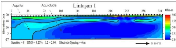
Gambar 4. Pemodelan Penampang 2D Lintasan 1
