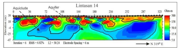
Gambar 17. Pemodelan Penampang 2D Lintasan 14
