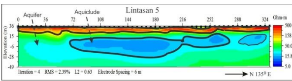
Gambar 8. Pemodelan Penampang 2D Lintasan 5
