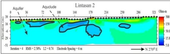
Gambar 5. Pemodelan Penampang Lintasan 2
