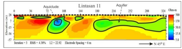
Gambar 14. Pemodelan Penampang 2D Lintasan 11
