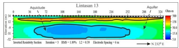
Gambar 16. Pemodelan Penampang 2D Lintasan 13
