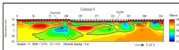
Gambar 11. Pemodelan Penampang 2D lintasan 8
