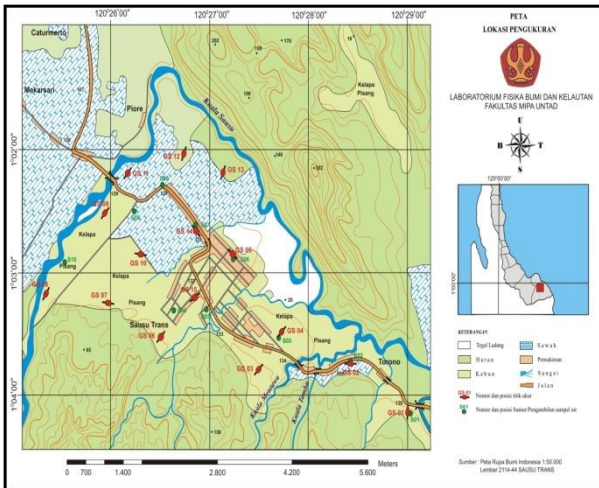
Gambar 2. Peta Lokasi Pengukuran
