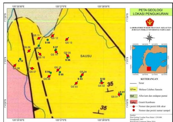
Gambar 3 Peta Geologi Lokasi Penelitian
