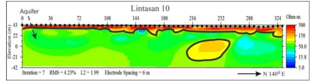
Gambar 13. Pemodelan Penampang 2D Lintasan 10
