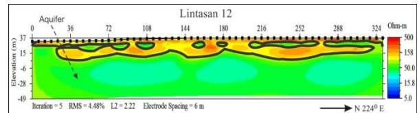
Gambar 15. Pemodelan Penampang 2D Lintasan 12
