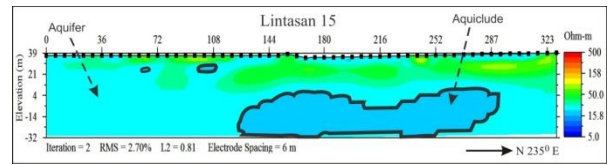
Gambar 18. Pemodelan Penampang 2D Lintasan 15
