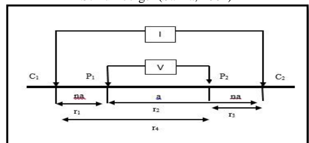
Gambar 1 Susunan Elektroda konfigurasiWenner-Schlumberger (Sakka, 2002)
